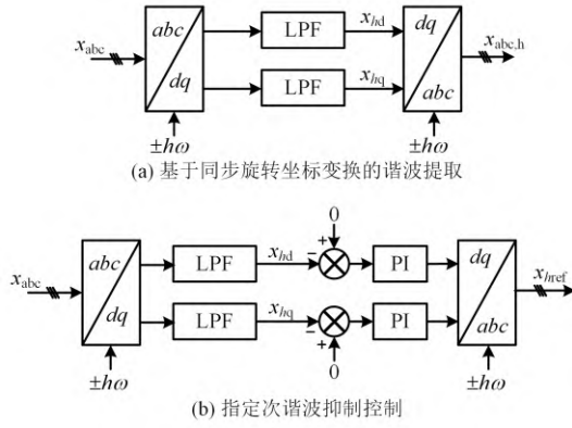
图 14 谐波电压抑制方法 Fig. 14 Harmonic voltage suppression method
