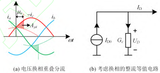
图 8 电压换相过程对直流电流的影响
