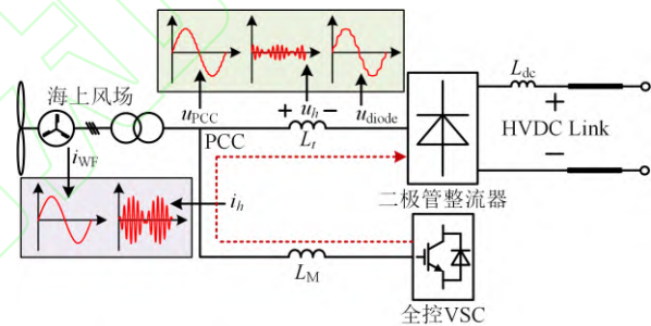
图 13 谐波电压抑制原理图
