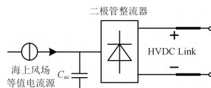
图 3 基于海上交流电流源和岸上直流电压源的简化等效模型
